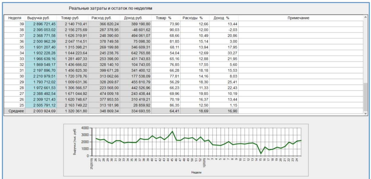
Рис. 10. Отчет «Анализ»
