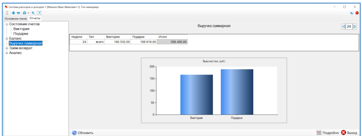
Рис. 7. Выручка суммарная
